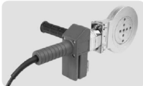
BOCAL DE TERMOFUSÃO
